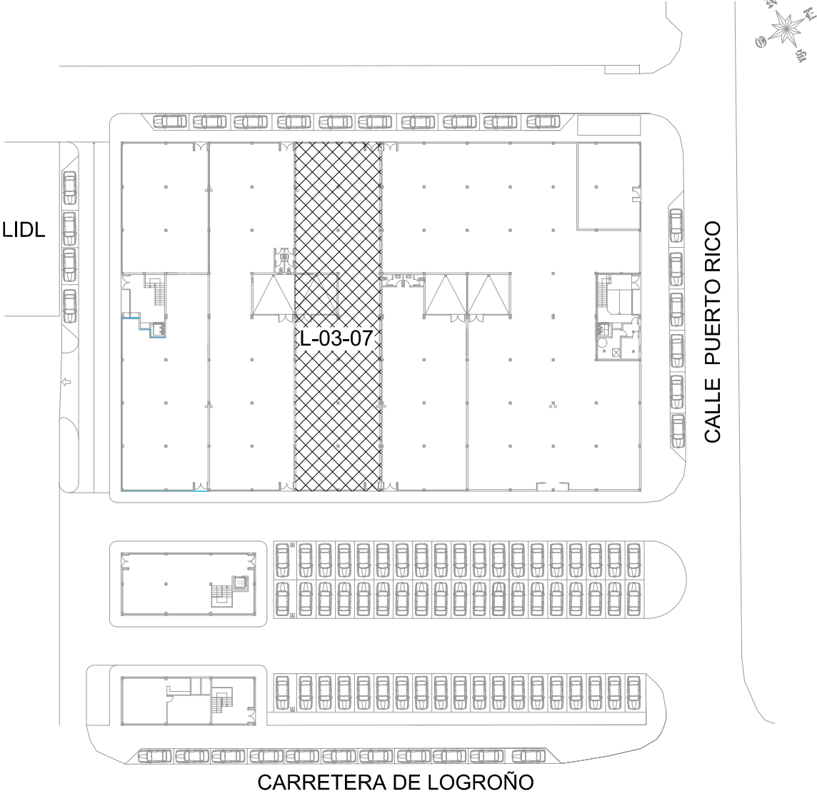
PLANTA BAJA (CONJUNTO LOCALES)
