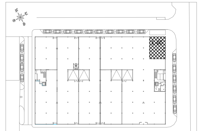
PLANTA BAJA (CONJUNTO LOCALES)
